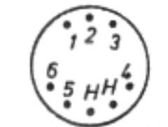
Sockelschaltung
